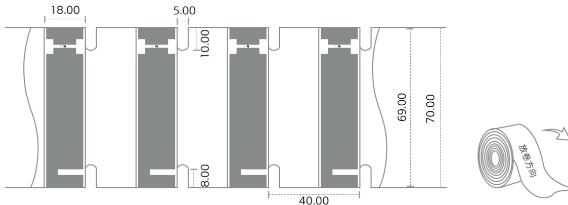
标签结构图
